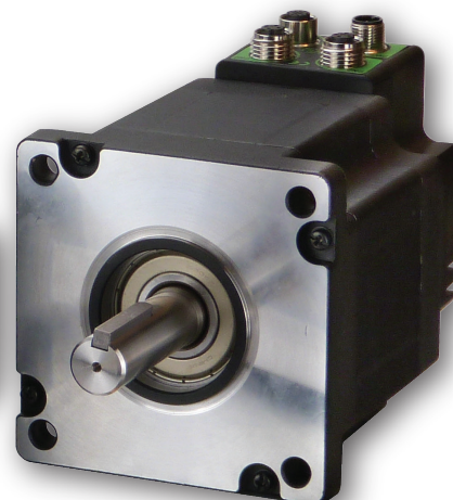
NEMA 43 (110 mm)
